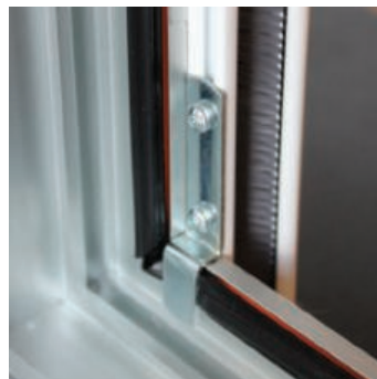
2 – Pose sur menuiserie Fixation sans perçage avec pattes métalliques
