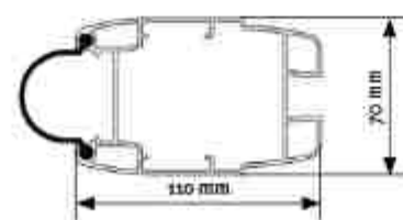
Montant - vue de dessus
