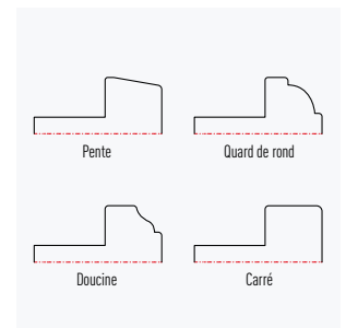
Moulures BOIS-ALU sur ouvrant possibles.
